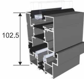
(D) Standard Threshold
